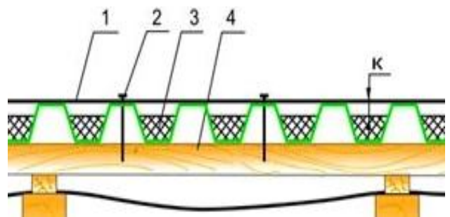
Рис. 10 Крепление конькового элемента
