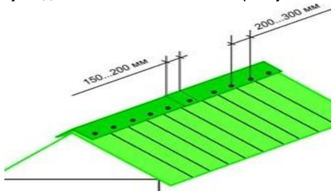
Рис. 10 Крепление конькового элемента
